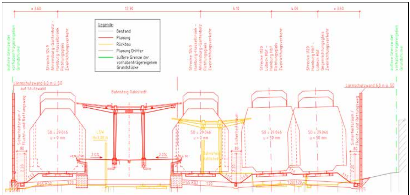
Grafik 1 DB-S4-Planung: Bahnstabsquerschnitt Rahlstedt, rechts die Fern-/Regionalbahngleise, links die S4-Gleise mit Bahnsteig
